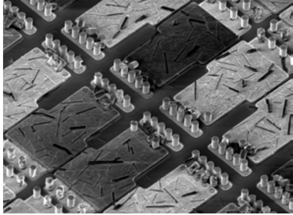
Vadné kondenzátory na křemíkovém čipu
